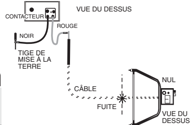
Figure 5. Récepteur de remise à zéro – Deuxième essai
