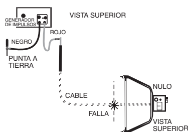
Figura 5. Receptor de Anulación – Segunda Vez
