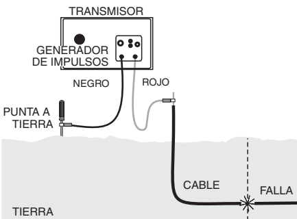
Figura 1. Instalación del Transmisor
